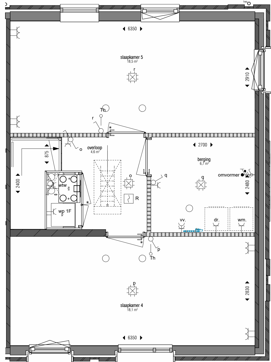
tweede verdieping 1:50
