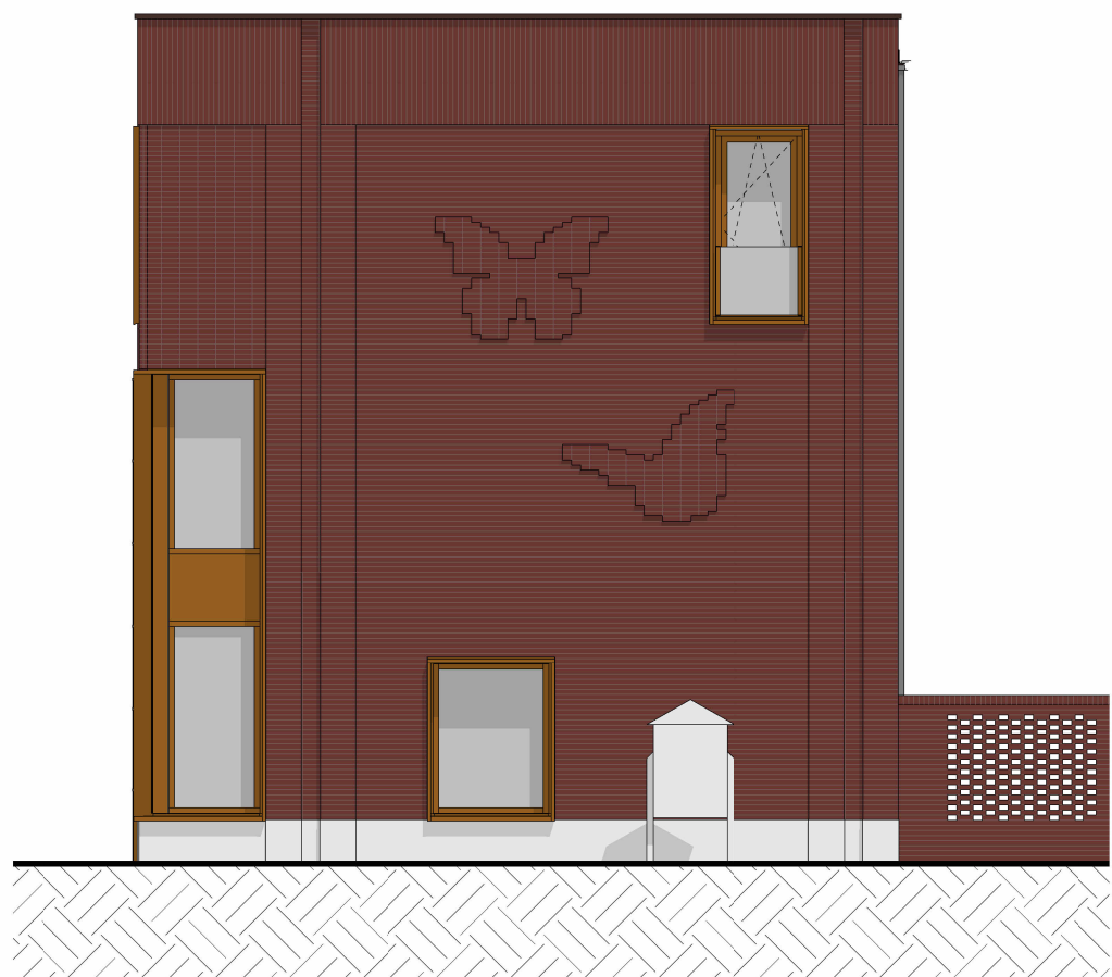
kopgevel 1:100
