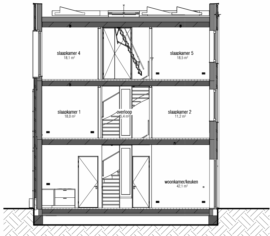
doorsnede 1:100
