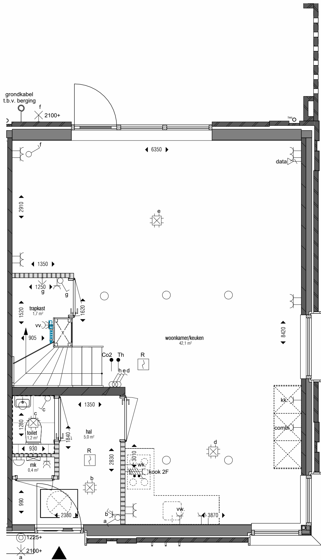
begane grond 1:50
