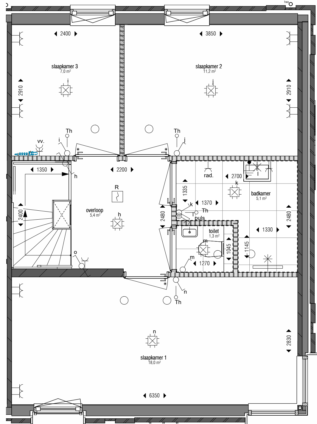
eerste verdieping 1:50
